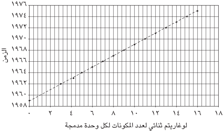
شكل ٢-٣: إعادة رسم لمخطط قانون مور. المصدر: منقول بتصريف من الأصل المنشور بمجلة «إلكترونيكس»، ٣٨ / ٨ (١٩ أبريل، ١٩٦٥).
